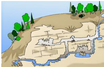
Schéma type d'un karst
